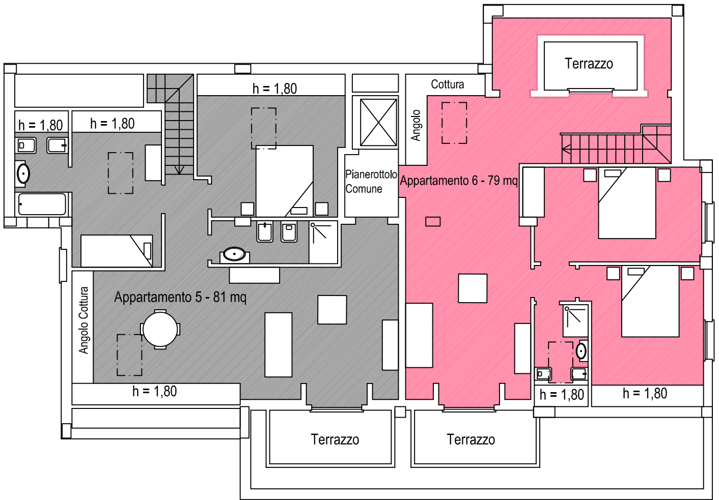
Piano Primo
